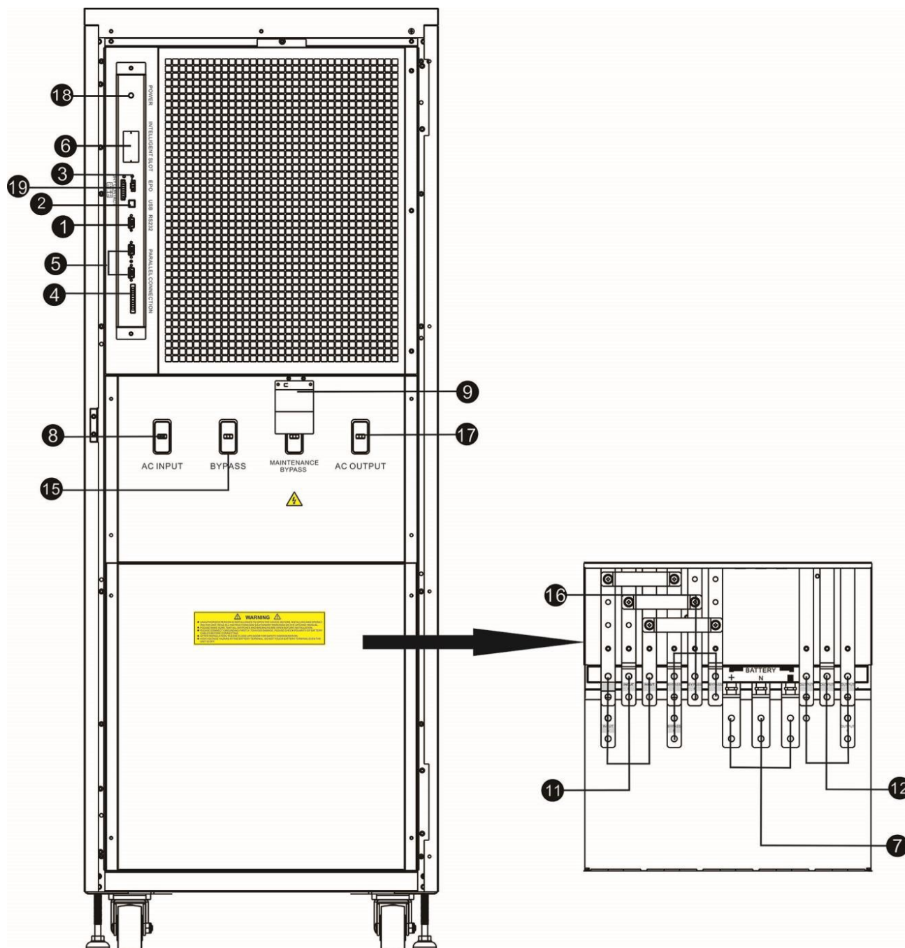
Вид спереди (при открытой двери) ИБП 100/120кВА
