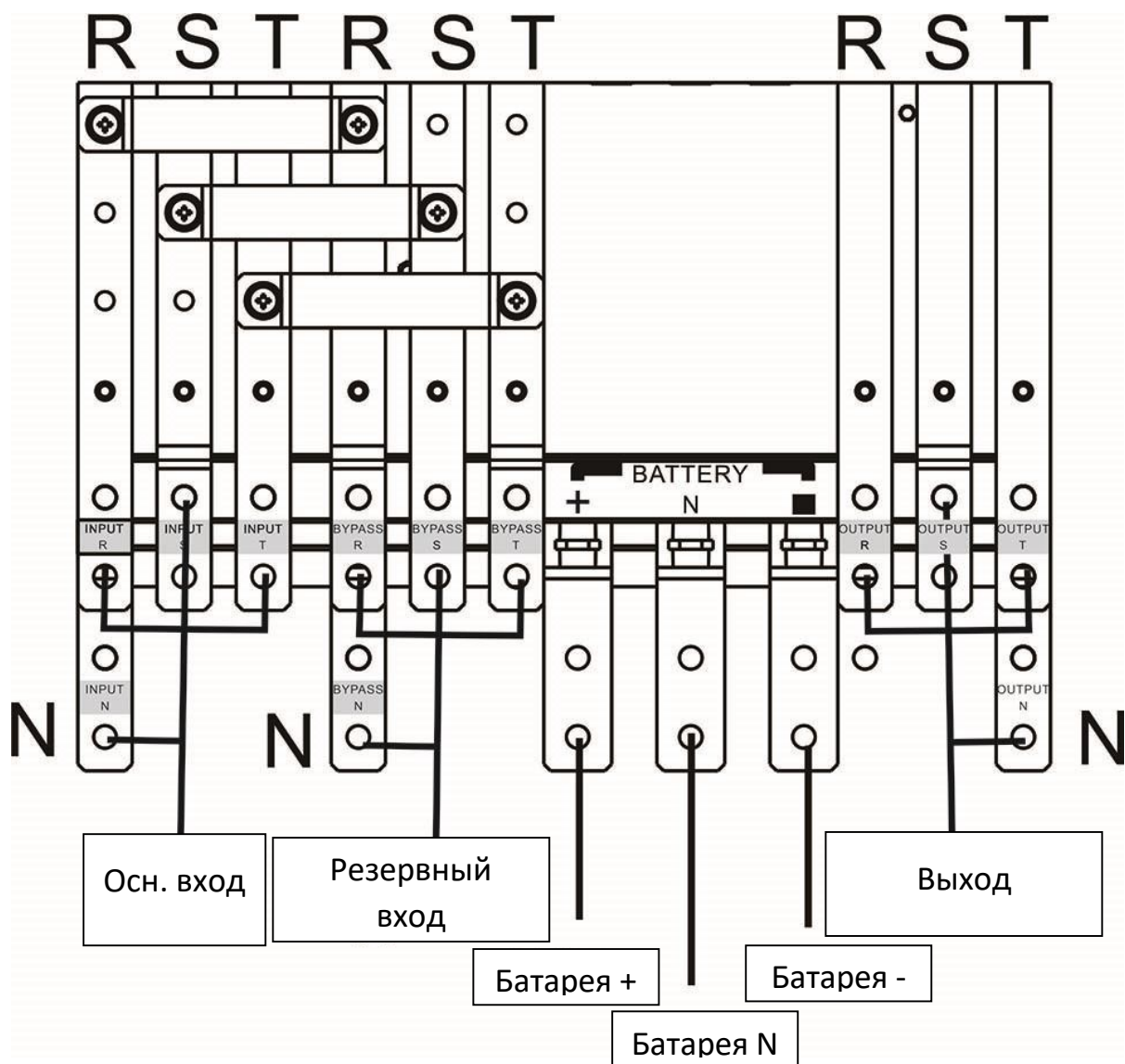
Подключение ИБП 100/120/180/200кВА
