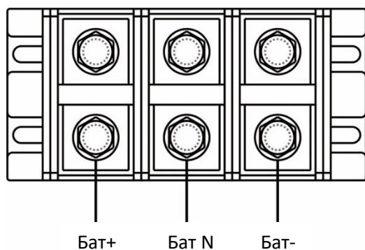
Подключение батарей ИБП 60кВА
