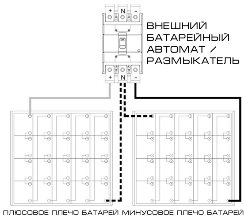
Внешний батарейный автомат / рубильник-разыкатель
