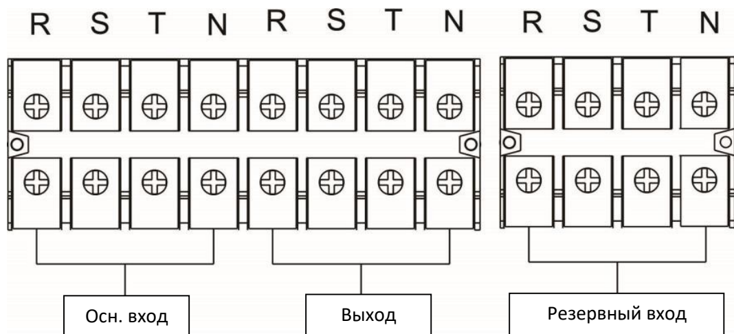
Подключение ИБП 60кВА
