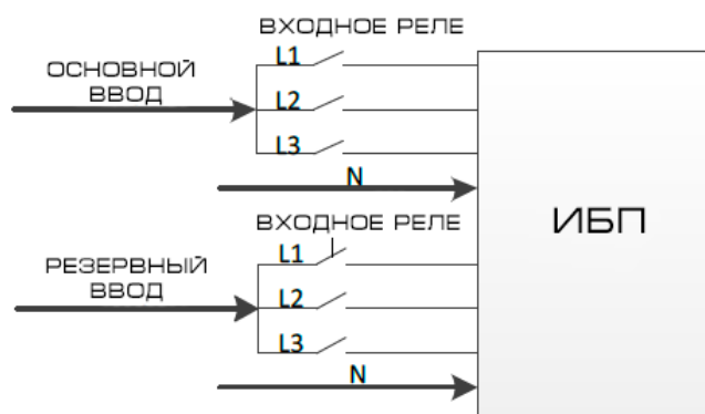
Входные реле ИБП
