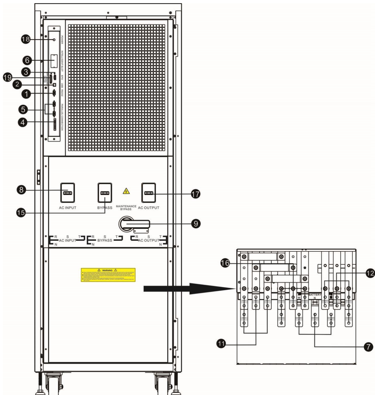
Вид спереди (при открытой двери) ИБП 180/200кВА
