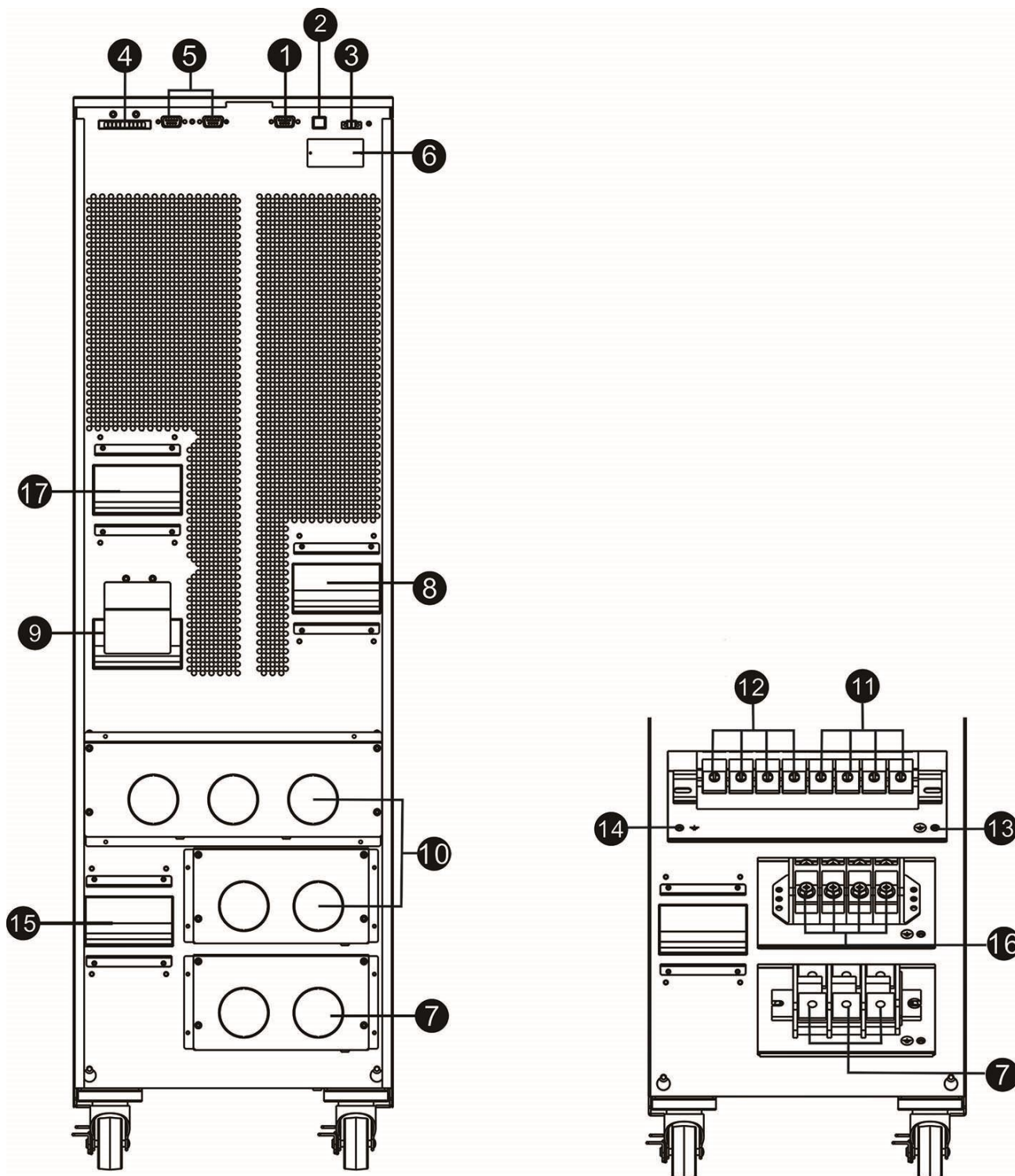
Вид сзади ИБП 60кВА
