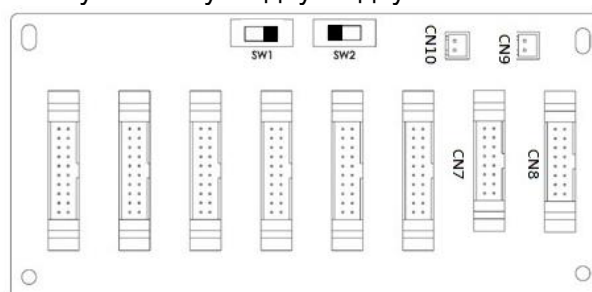
Плата параллельной работы ИБП 2.
