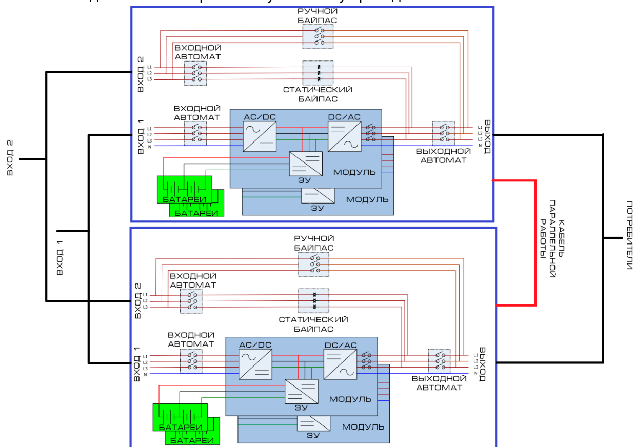
Подключение двухфидерных ИБП в параллельную систему.
