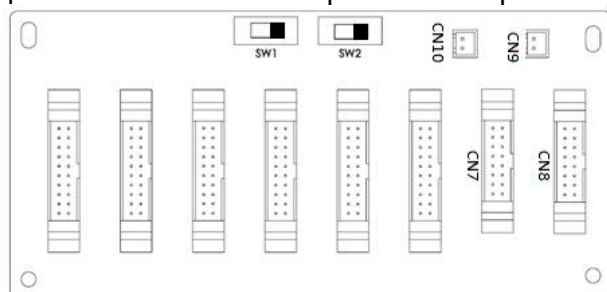
Плата параллельной работы ИБП 1.
