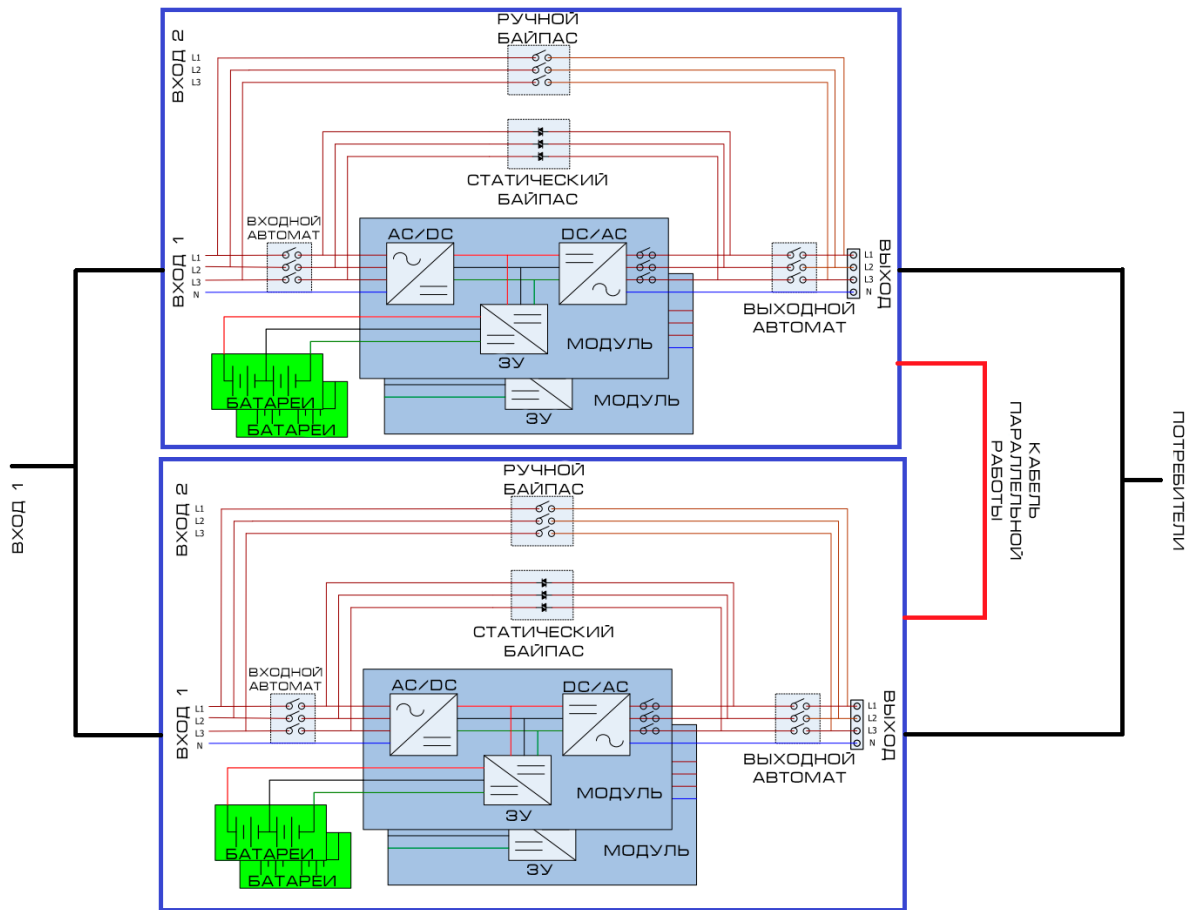
Подключение однофидерных ИБП в параллельную систему.
