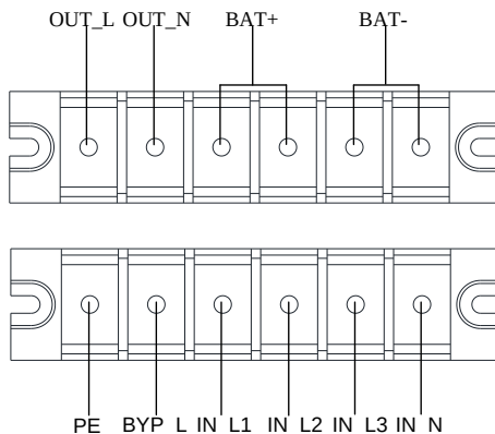
Клеммы подключения ИБП 20кВА 3/1
