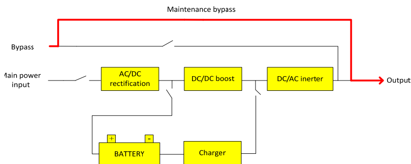
Рисунок 1.6 Схема рабочего процесса в режиме ручного Байпаса.
