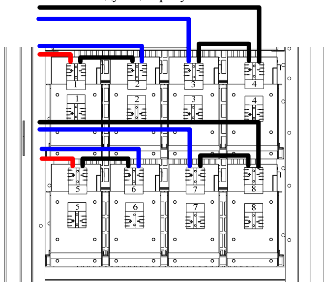
Рисунок 2.15 Схема подключения батарейного блока
