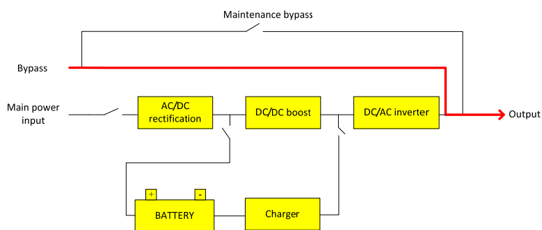
Рисунок 1.5 Схема рабочего процесса в режиме электронного Байпаса.
