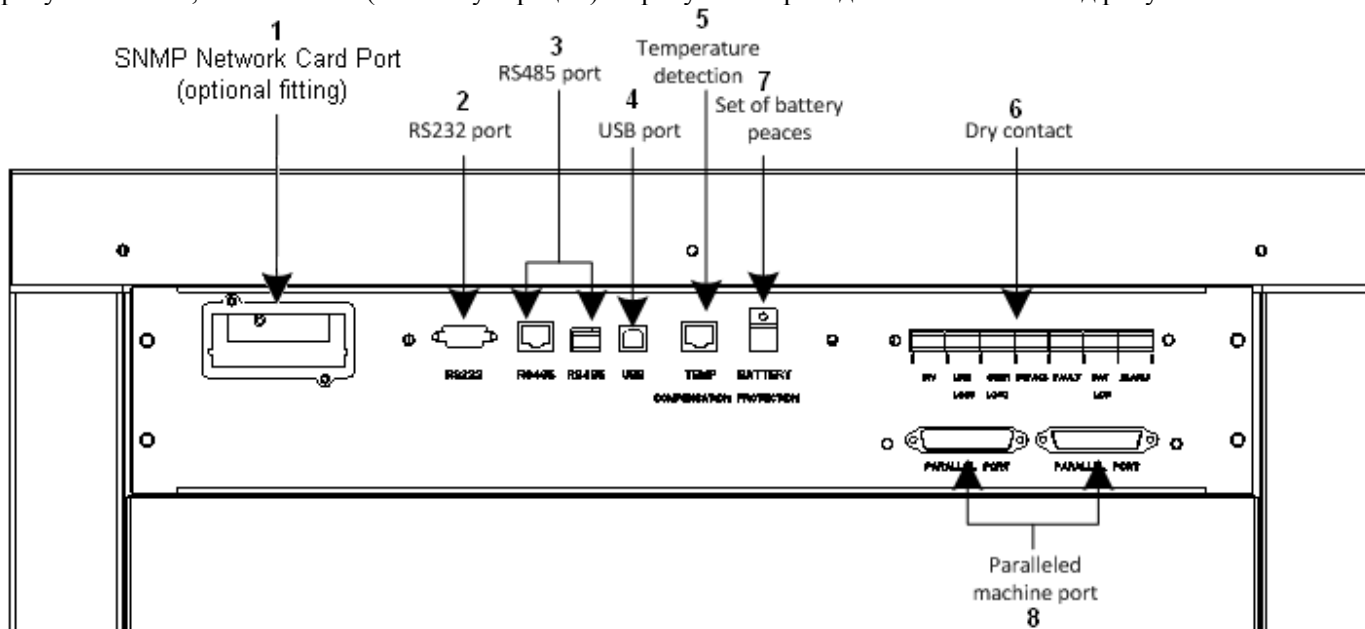
Рисунок 1. Коммуникационные порты ИБП Power-Vision Black HF 10-60кВА
