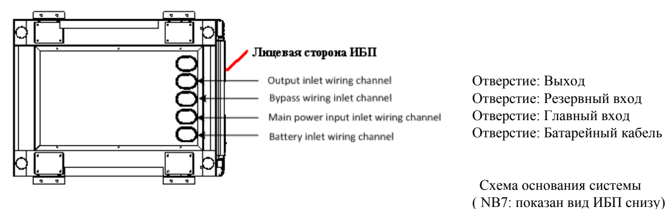
Рисунок 2.8 Входные и выходные кабельные каналы ИБП Power-Vision Black HF (10-60кВА)
