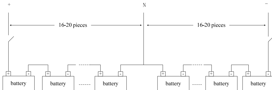
Рисунок 2.12 Схема подключения батарей
