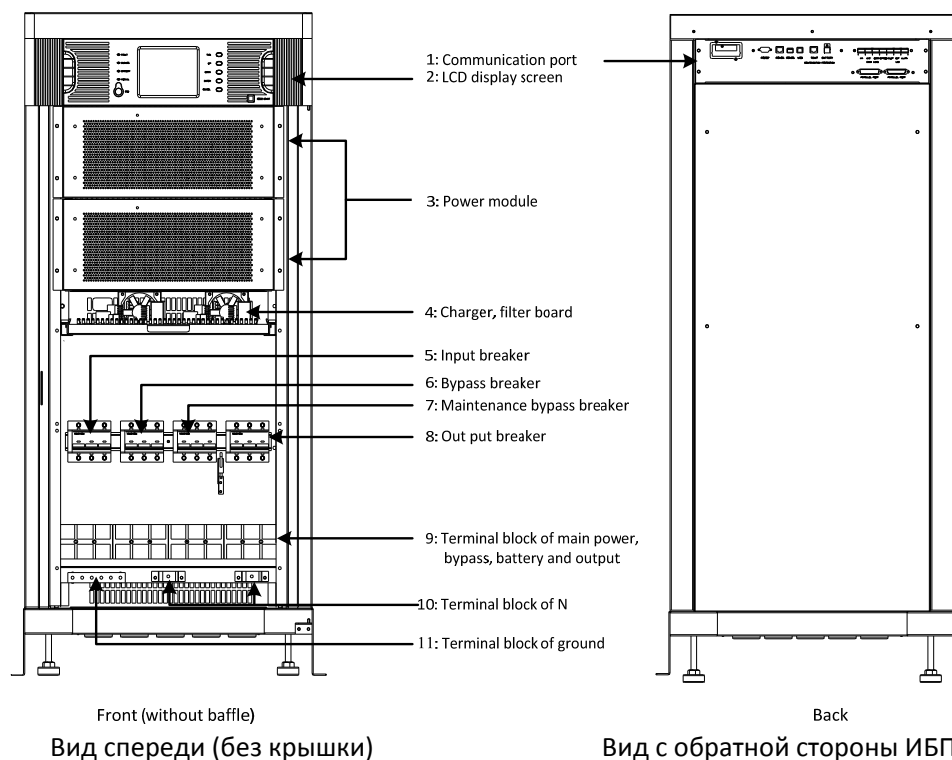
Рисунок 1.2 Структура PowerVisionBlack HF 40-60кВА
