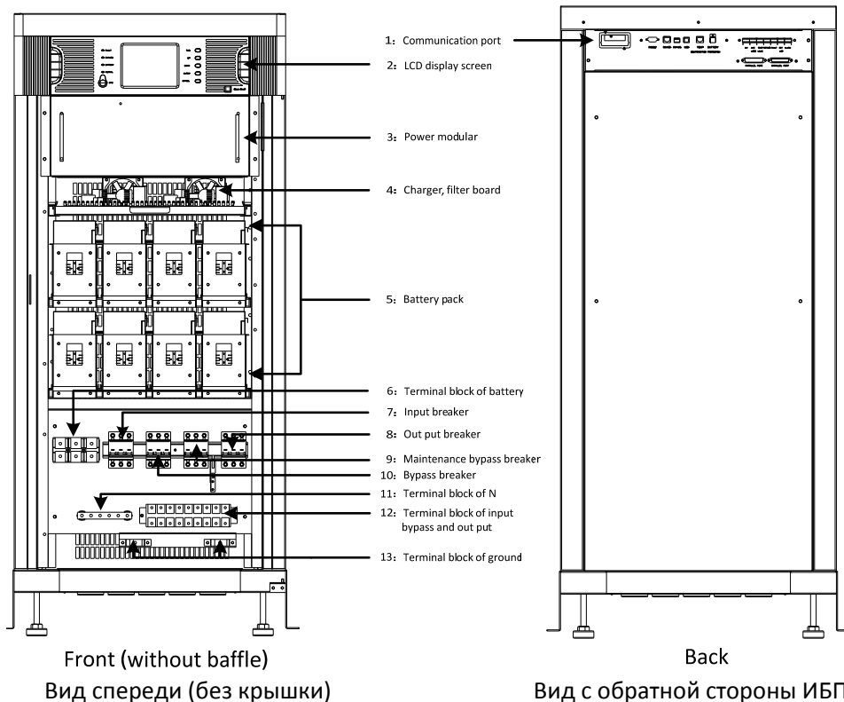
Рисунок 1.1 Структура PowerVisionBlack HF 10-30кВА
