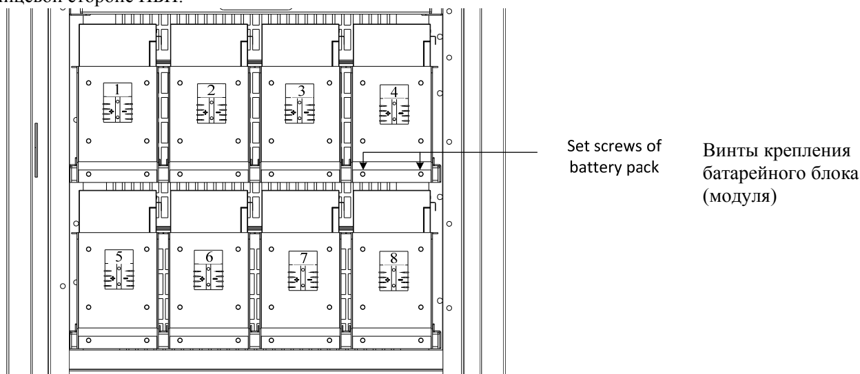
Рисунок 2.13 Батарейный блок
