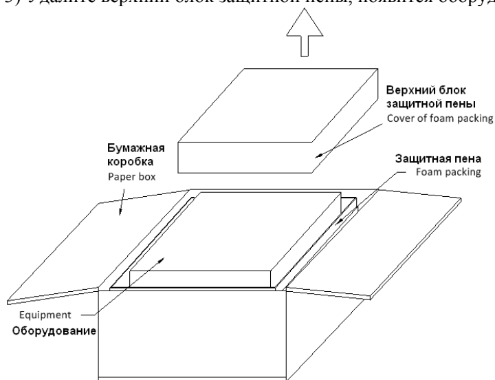
Рисунок 2.6 Извлечение модулей
