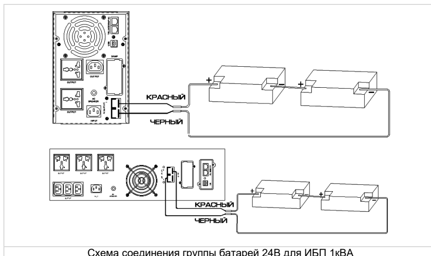
Схема соединения группы батарей 24В для ИБП 1кВА
